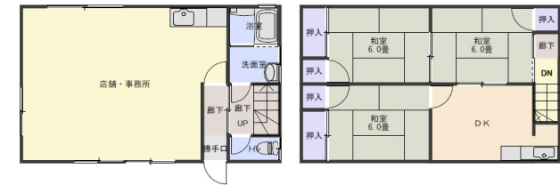
1階 縮尺 1/100
